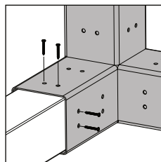
Detalle A
